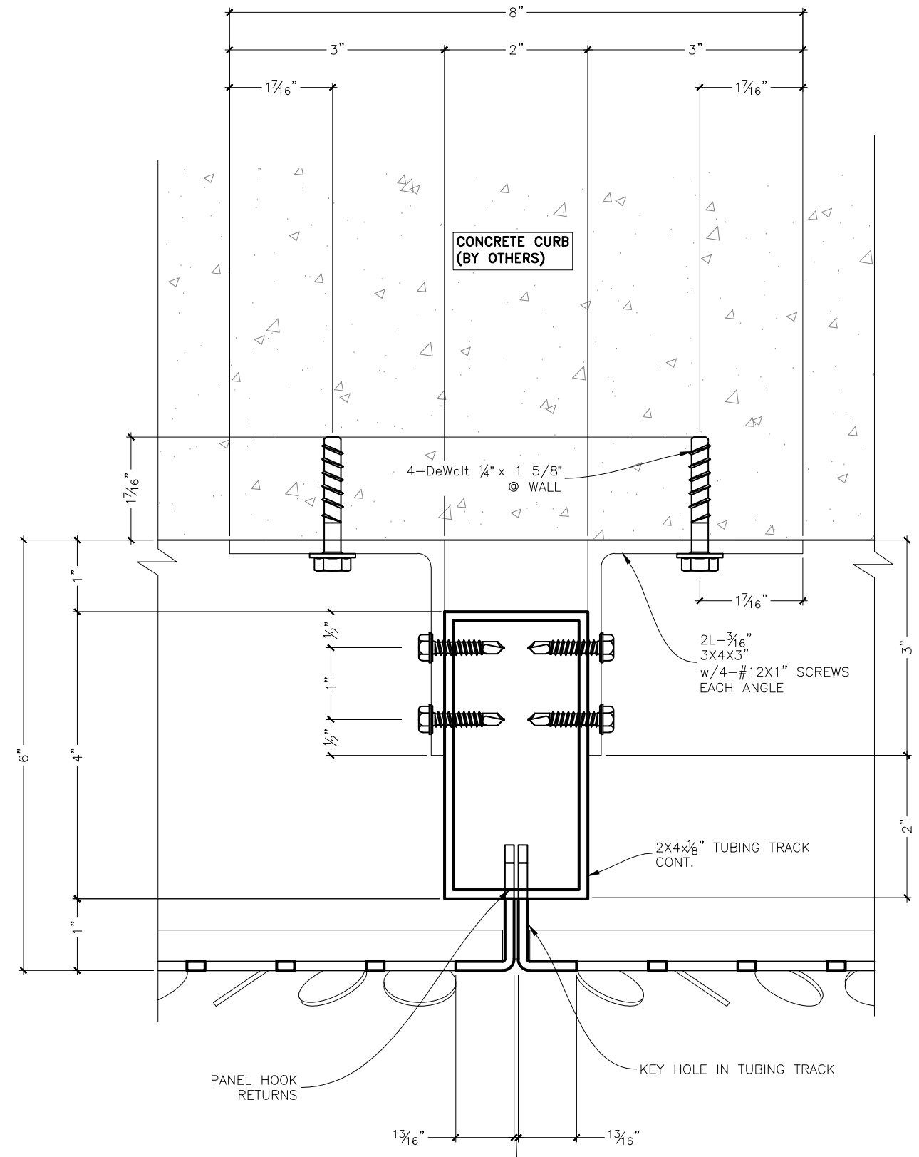
2 DETAIL D1 SCALE 6"=1'-0" SCB REF.: N/A
